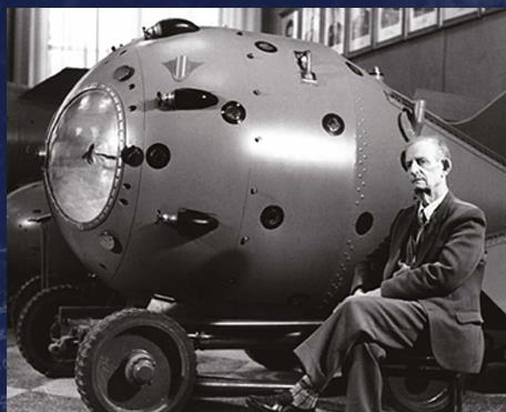
Академик Ю.Б. Харитон рядом с корпусом первой советской атомной бомбы РДС-1
