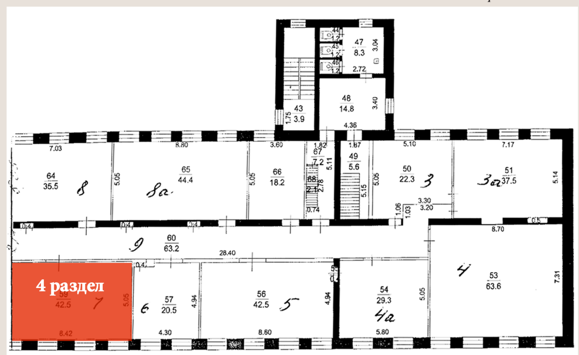
план второго этажа
